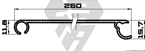
АДАПТЕР ПОВОРОТНЫЙ УНИВЕРСАЛЬНЫЙ
