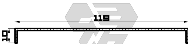
ЗАГЛУШКА Т-СОЕДИНЕНИЯ СТОЕК
