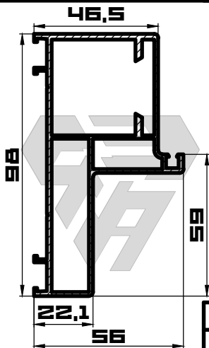
РАМА ДЛЯ СКРЫТЫХ НАВЕСОВ
