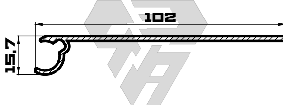
АДАПТЕР ПОВОРОТНЫЙ 90-1102ММ
