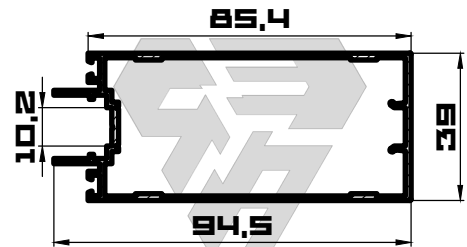
СТОЙКА ОДИНАРНОГО ОСТЕКЛЕНИЯ
