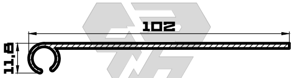
АДАПТЕР ПОВОРОТНЫЙ 90-2 102ММ
